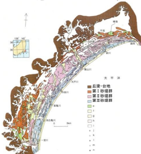
九十九里浜の浜堤 森脇 孝弘(1979)
