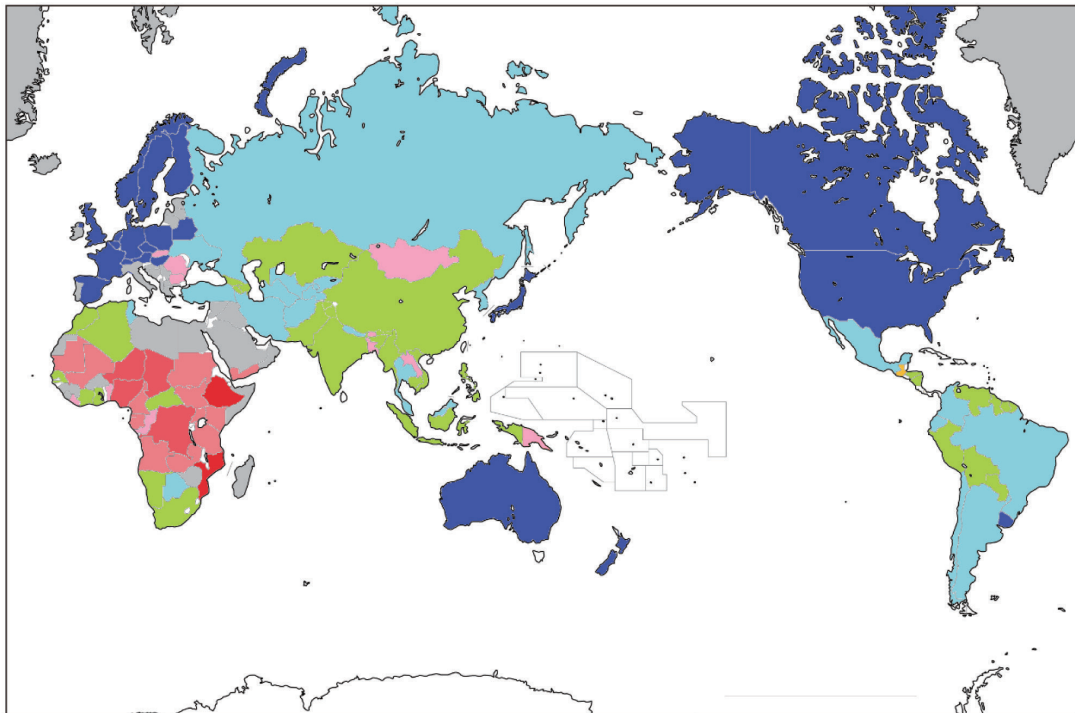
【図 安全に管理された飲み水を利用できる人の割合 2020】
